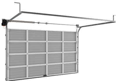
Секционные ворота из однослойных панелей с торсионным механизмом RSD02 SLP
